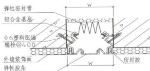
单列嵌平型
