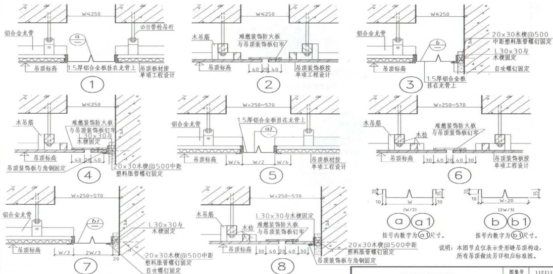
吊顶变形缝
