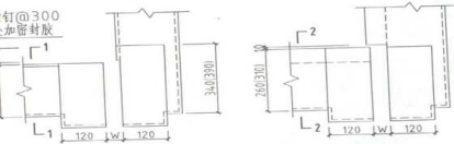
⑤ 女儿墙顶部平面 (未加盖板,压顶无挑出)
