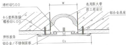
金属盖板型
