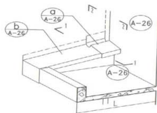
① 加金属盖缝板后示意图
