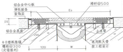
双列嵌平型
