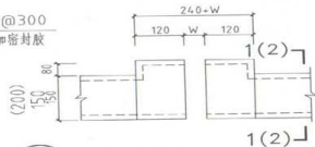
⑤ 女儿墙顶部平面 (没加盖板)
