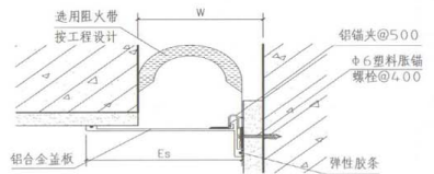
金属卡锁型
