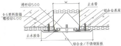
金属盖板型
