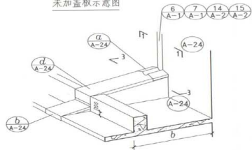
③ 加金属盖板后示意图
