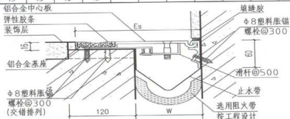
双列嵌平型
