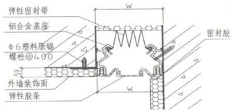
单列嵌平型
