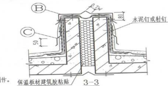
块瓦坡屋面变形缝(二)
