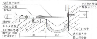
金属卡锁型
