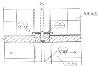
① 女儿墙(外天沟)平面
