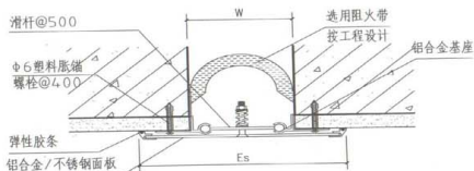
抗震型
