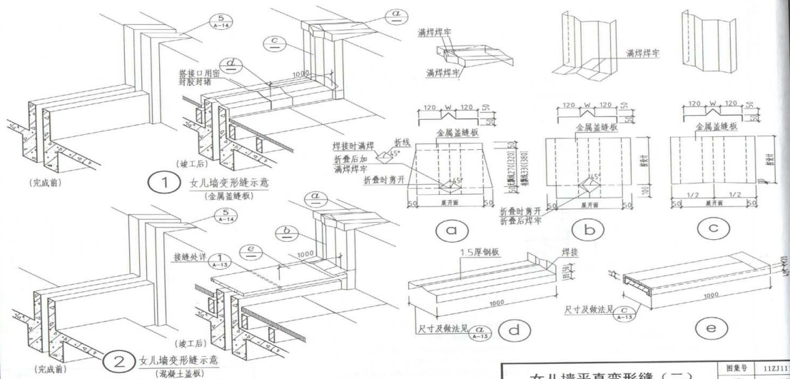
女儿墙平直变形缝 (二)
