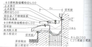
金属盖板型
