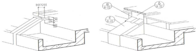
B 外天沟平直变形缝示意
