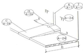
② 加金属盖板后示意图
