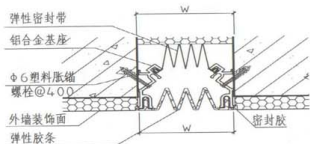
单列嵌平型
