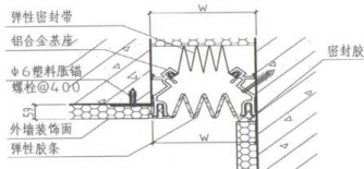
单列嵌平型
