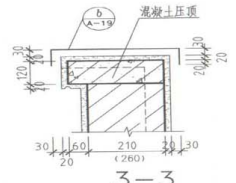
3-3 (压顶有挑出)
