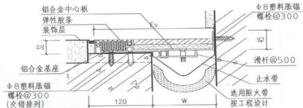
双列嵌平型
