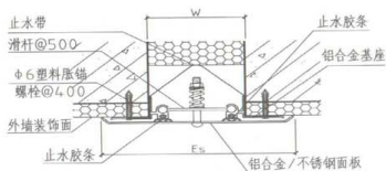
抗震型
