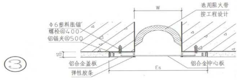
金属卡锁型
