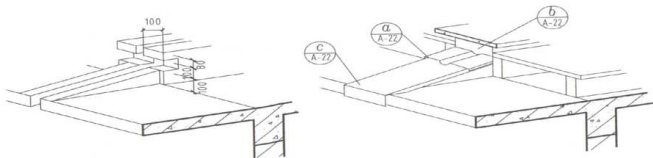
(未加盖板) A 挑檐平直变形缝示意
