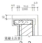
2-2 压顶有挑出
