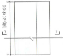
3—3 剖面
