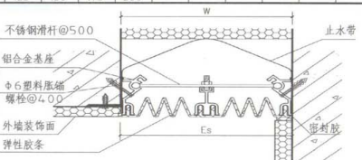
单列嵌平型
