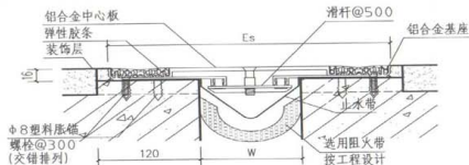
双列嵌平型
