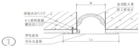
金属卡锁型
