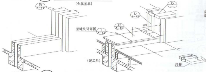
② 女儿墙(压顶无挑出)变形缝示意 (混凝土盖板)
