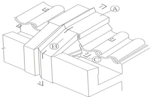
① 檐口变形缝与块瓦坡屋面相接处理
