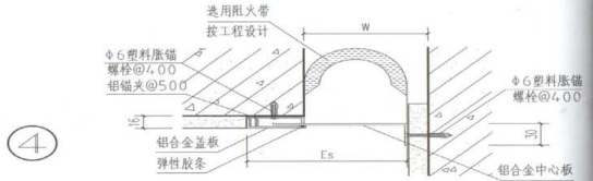
金属卡锁型
