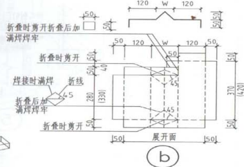
女儿墙转角变形缝(二)
